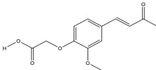
Слика 5. Енон 1 ( (E) -2- (2-метокси-4- (3-оксобут-1-ен-1-ил) фенокси) ацетат
