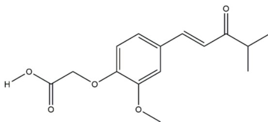
Слика 6. Енон 2 ( (E) -2- (2-метокси-4- (4-метил-3-оксопент-1-ен-1-ил) фенокси) ацетат
