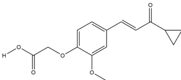
Слика 8. Енон 4 ( (E) -2-(3-циклопропил-3-оксопроп-1-ен-1-ил)-2-метоксифенокси) ацетат
