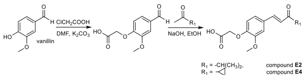
Слика 14. Синтеза енона E2 и E4
