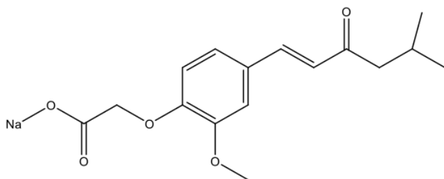
Слика 11. Со Енона 3 Натријум (E)-2- (2-метокси-4- (5-метил-3-оксхекс-1-ен-1-ил) фенокси) ацетат ( M_r = 314,31 \text{ g/mol} )
