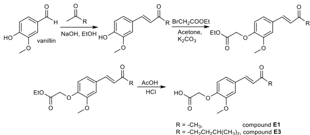
Слика 13. Синтеза Енона E1 и E3
