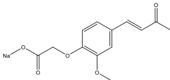
Слика 10. Со Енона 2 Натријум (E)-2- (2-метокси-4- (4-метил-3-оксопент-1-ен-1-ил) фенокси) ацетат ( M_r = 300,29 \text{ g/mol} )
