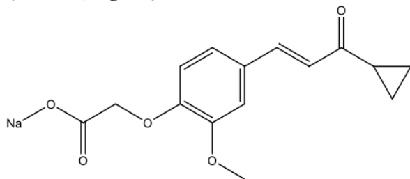
Слика 11. Со Енона 3 Натријум (E)-2- (2-метокси-4- (5-метил-3-оксхекс-1-ен-1-ил) фенокси) ацетат ( M_r = 314,31 \text{ g/mol} )
