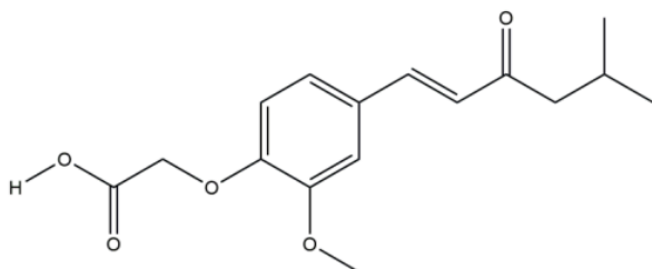
Слика 7. Енон 3 ( (E) -2- (2-метокси-4- (5-метил-3-оксхекс-1-ен-1-ил) фенокси) ацетат
